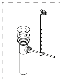
Montaje del drenage
