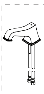
Montaje del surtidor
