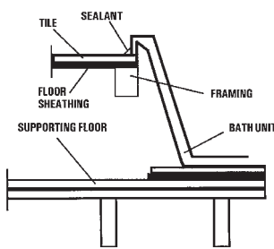
1E Sunken Installation
