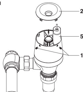
Fig. 11a PILE NORMALE
