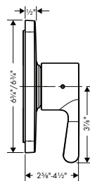
AXOR Citterio M 34808xx1
