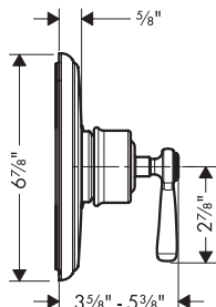
AXOR Montreux 16508xx1
