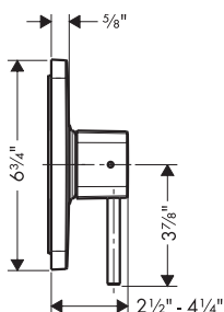
AXOR Urquiola 11408xx1
