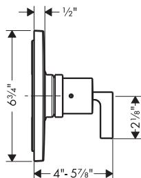
AXOR Citterio 39414xx1
