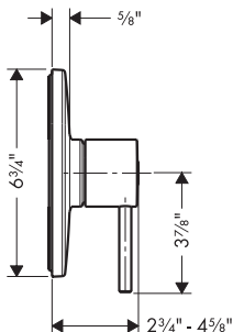
AXOR Uno 38418xx1
