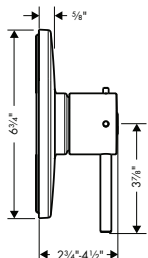
AXOR Starck 10407xx1
