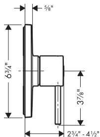
AXOR Massaud 18978xx1
