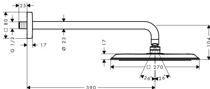
AXOR Citterio C 270/270 1jet 28790XX0/28791XX0
