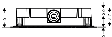
AXOR Citterio C 270/270 1jet 28794XX0/28795XX0
