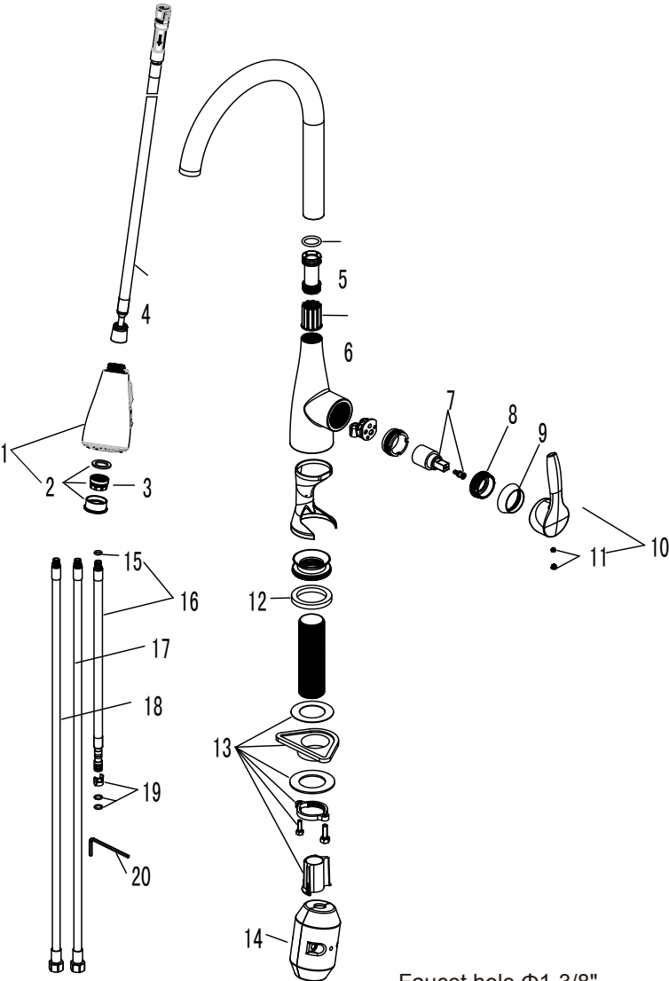
Faucet hole Φ1-3/8"
