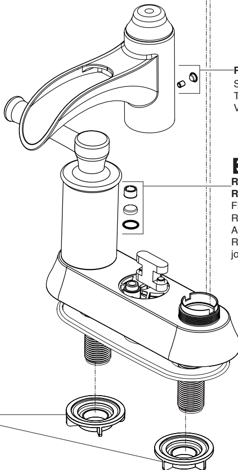
RP6183 Locknuts Contratuercas Écrous de Blocage
