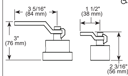
HW75P32-▲ Wheel Handle
