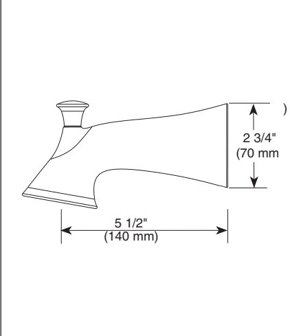
RP51303 ▲ (Pull-Up Diverter)
