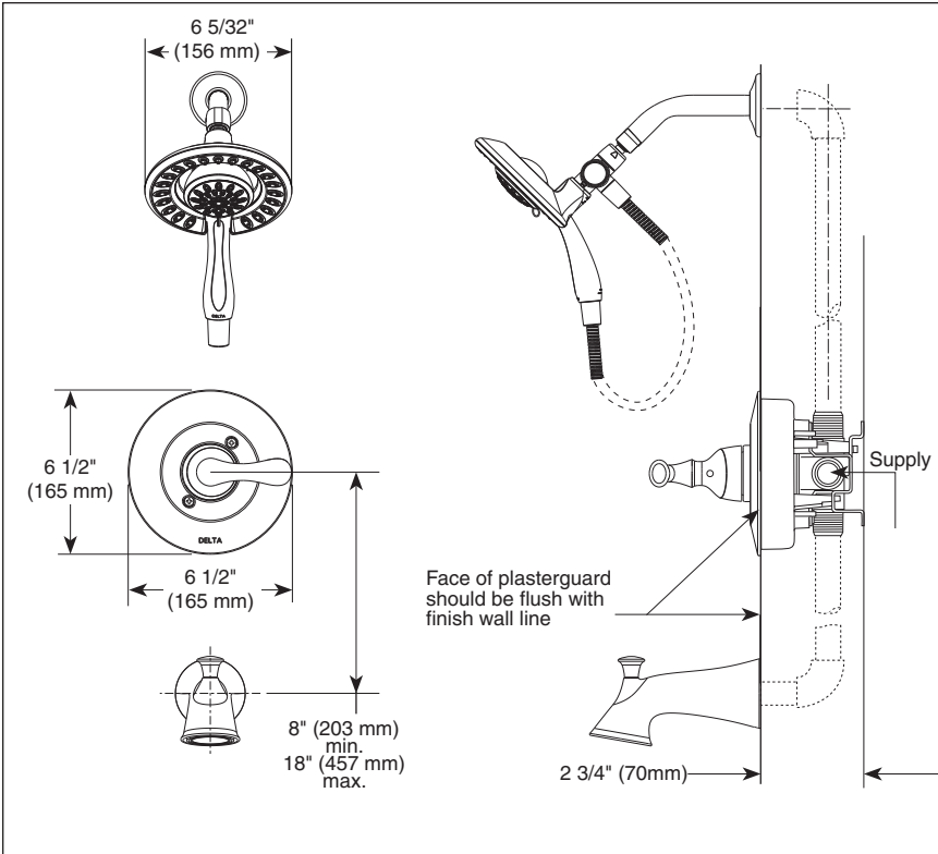
RP51303 ▲ (Pull-Up Diverter)
