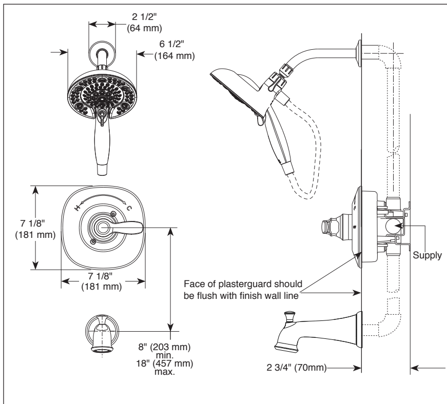
RP52153▲ (Pull-Up Diverter)
