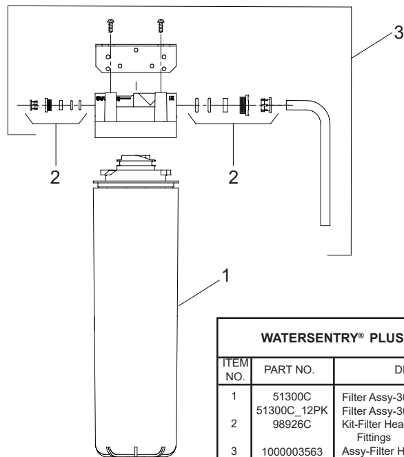
FIG. 13 Water Filter Exploded View Filtro de agua despiece Vue éclatée de l'eau filtre
