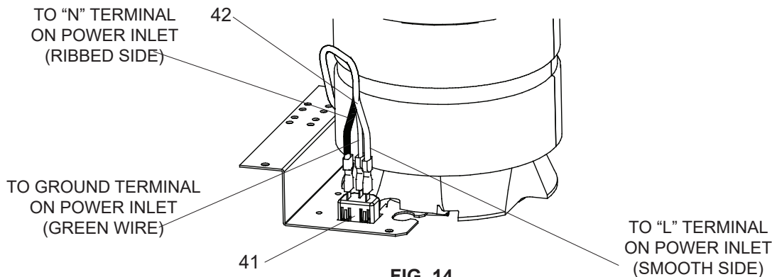
FIG. 14 220V/240V Power Inlet Detail 220V/240V potencia entrada detalle 220V/240V alimentation détail
