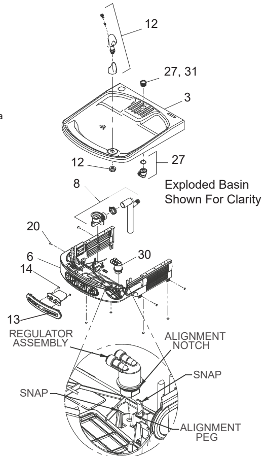
Fig. 6 EZ/LZ Right Hand Unit
