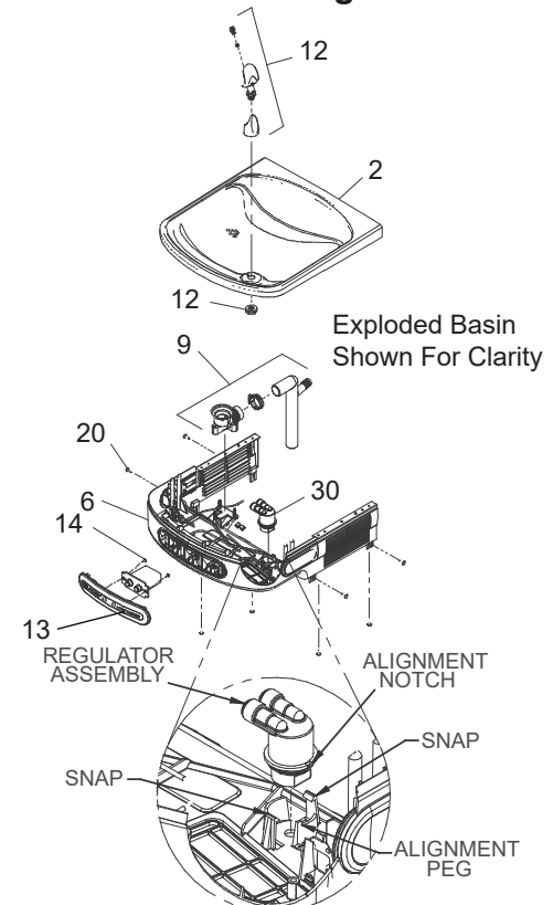
Fig. 7 EZ/LZ Left Hand Unit
