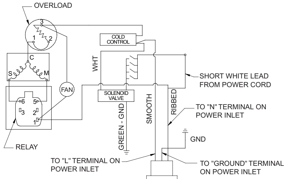
Fig. 8 220V Wiring Diagram Esquema eléctrico 220V Diagramme de câblage 220V
