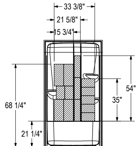
OPTIONNAL REINFORCEMENT (Back Wall)
