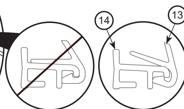
SETTING BLOCK INSTALLATION INSTALLATION DU GUIDE DE PANNEAU INSTALACION DE LA GUÍA DEL PANEL
