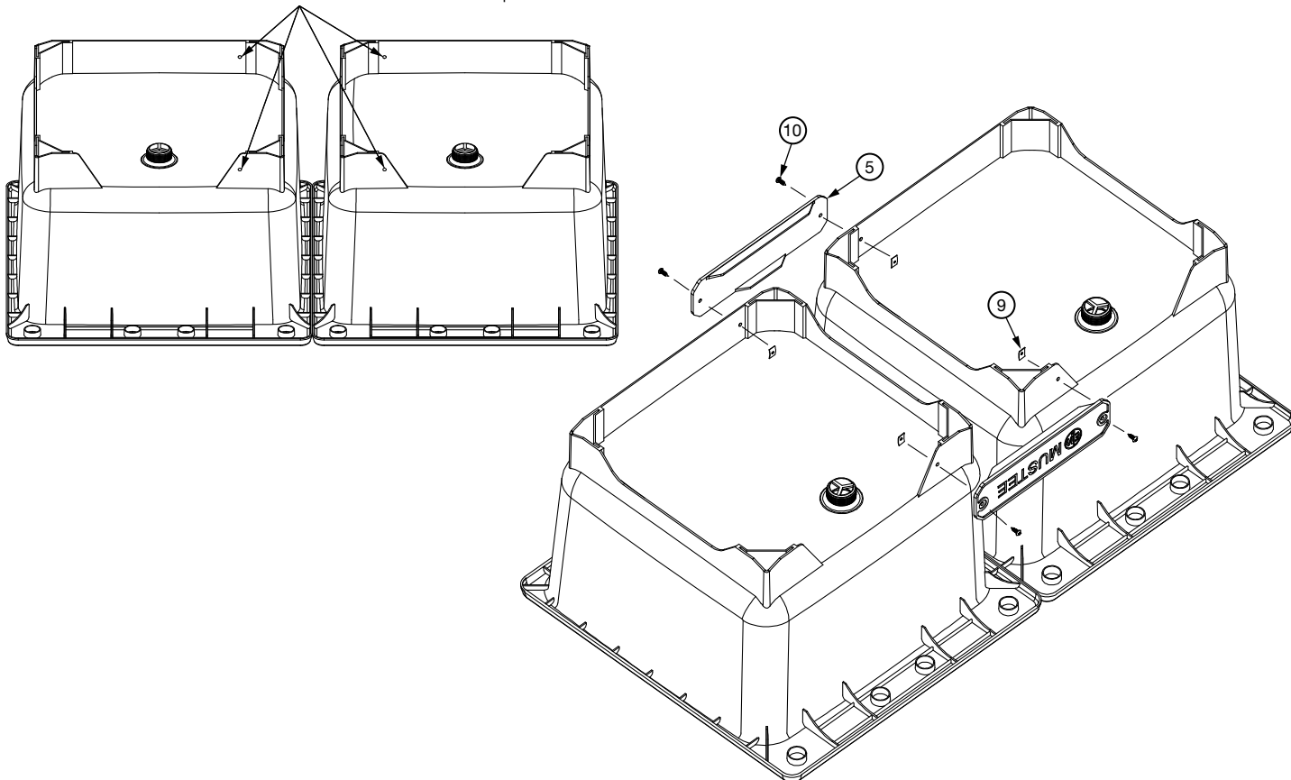
Drilled Holes Orificios • Trous percés
