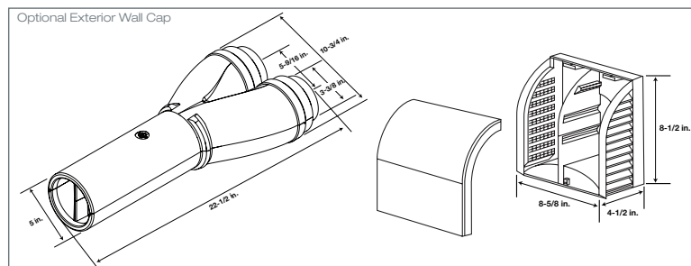
FV-WC04VE1
