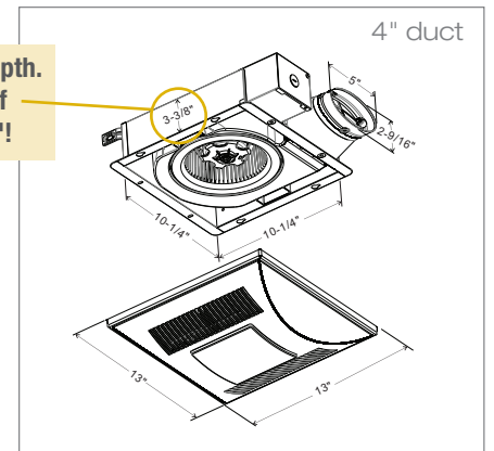
FV-08/10VSL3E
