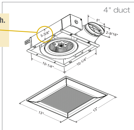
FV-05/08/10VS3E
