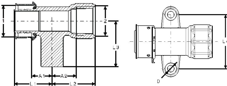
PEX Press Fire Sprinkler Adapter
