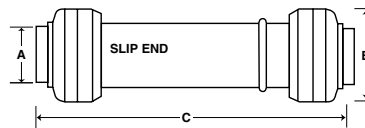
Slip Coupling* Dimensions
