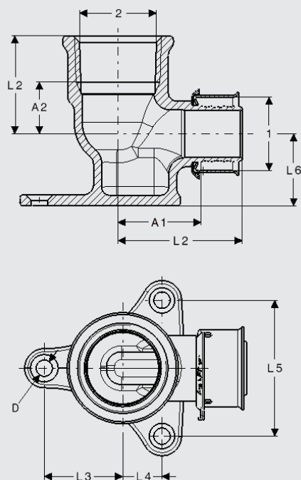
PEX Press Fire Sprinkler Elbows
