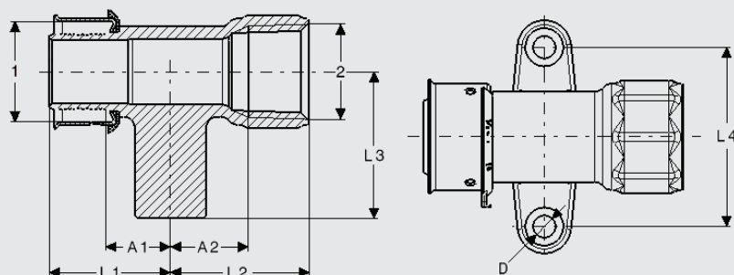
PEX Press Fire Sprinkler Adapter
