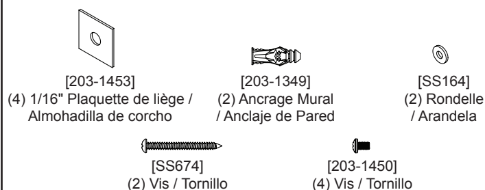
[216-1184] Sac de visserie / Bolsa de herrajes
