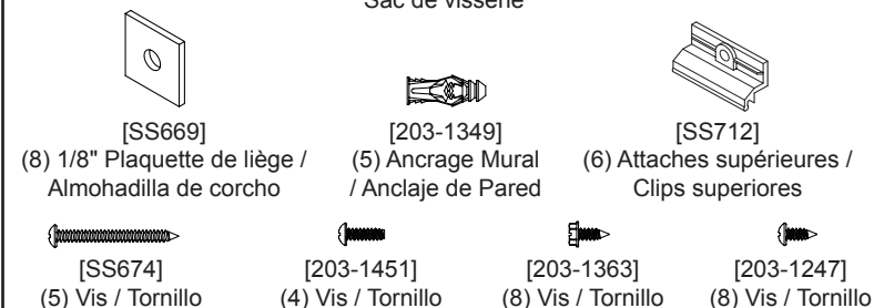
[216-1183] Sac de visserie / Sac de visserie
