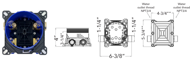
Forever Box SMSUB
