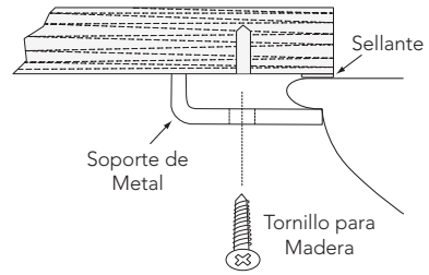
Llanta estándar
