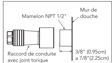
Raccord de Conduite avec Joint Torique
