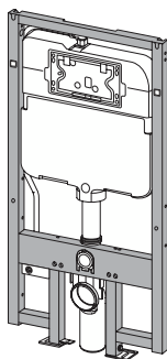
Réservoir Mural
